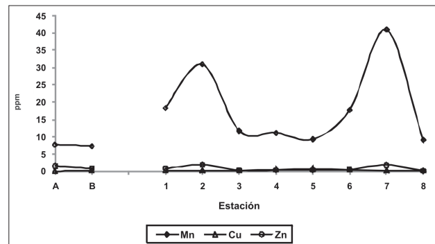
Figura 4b - Análisis de Manganeso (Mn), Cobre (Cu) y Zinc (Zn) de los suelos manglar en las estaciones de las localidades muestreadas en el Horizonte B.
